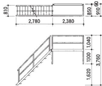
SH-HP型/階段
