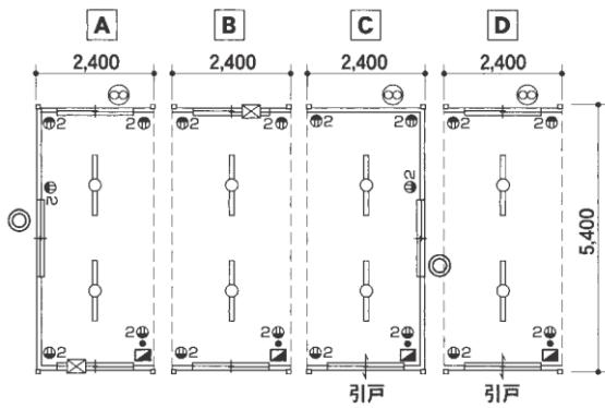
SH-HP72 平面図
